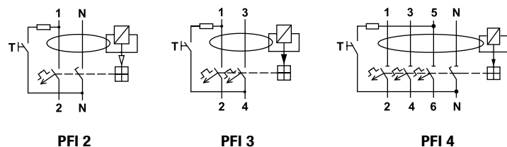
Schéma zapojení
