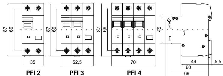
Rozměrový náčrt PFI 2, PFI 3 a PFI 4
